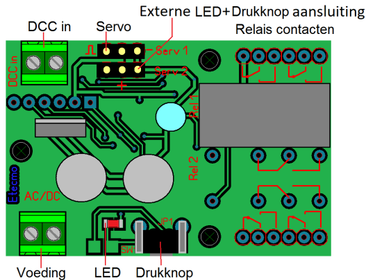
Overzicht van de aansluitingen van de servo decoder.
