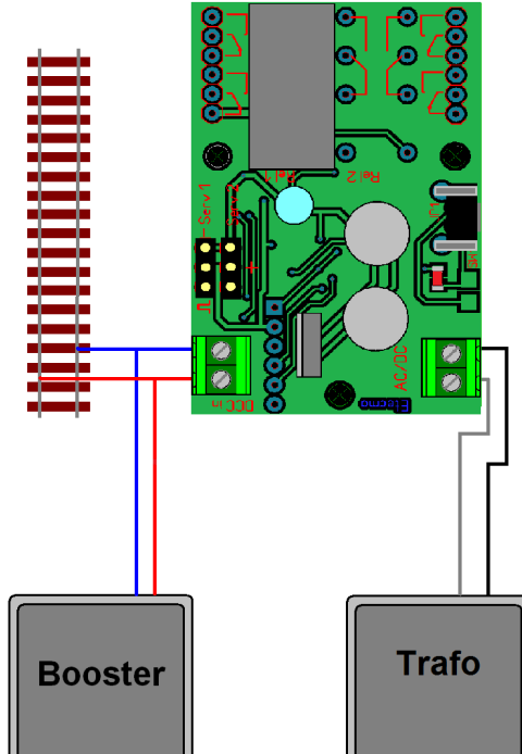
Aangesloten met een aparte voedingsbron.
